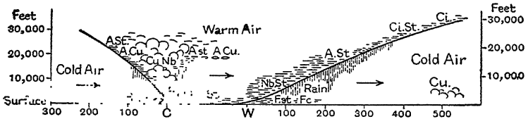
चित्र ५१ (a) — उष्णखंड में चक्रवात में बादल और मौसम
